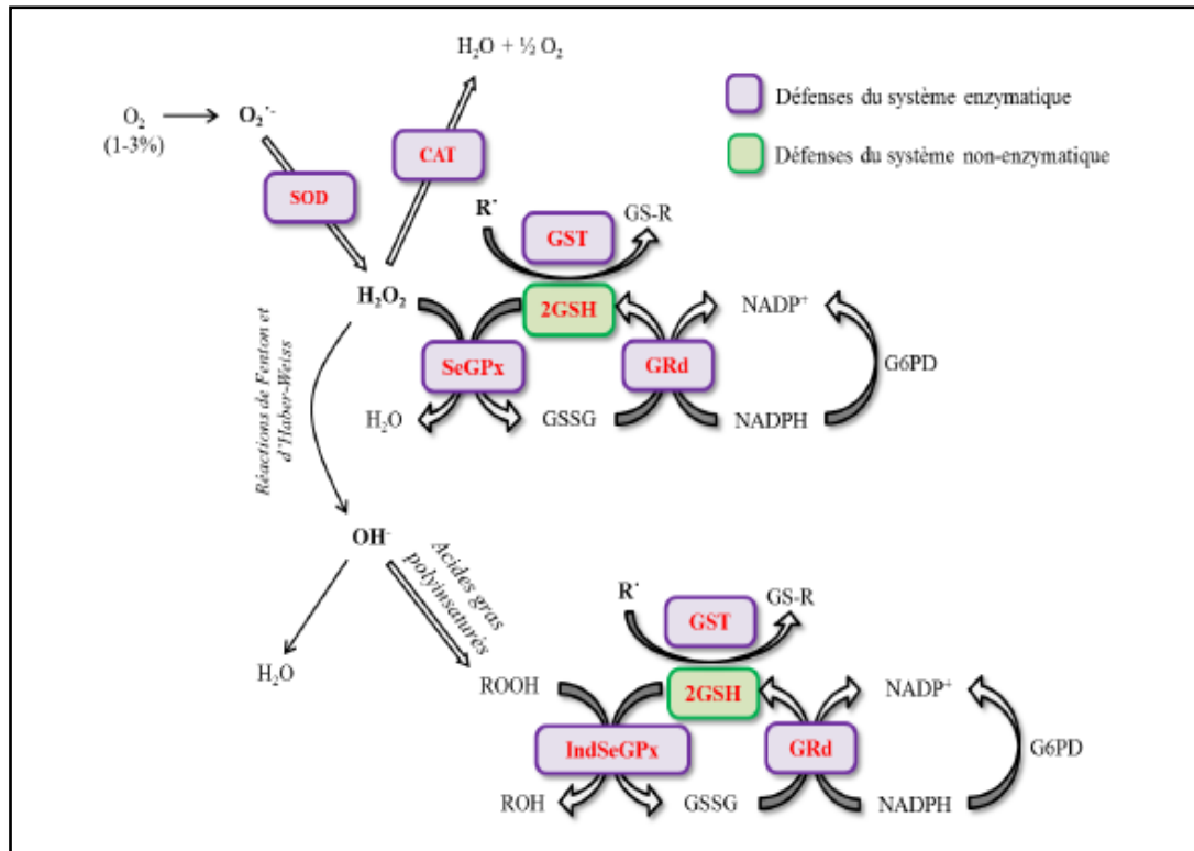
Figure 13. Schéma des systèmes enzymatiques et non-enzymatiques de détoxification des ROS.
