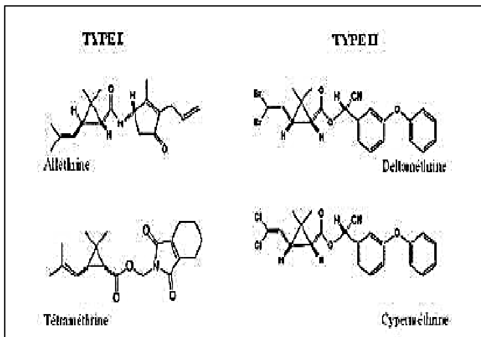
Figure 1. Exemples des insecticides appartenant aux types I et II des pyréthrinoïdes (Gasmi, 2018).
